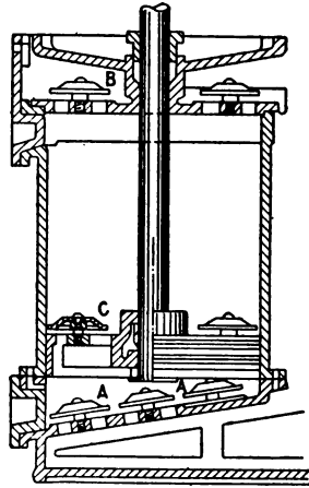
FIG. 16.—U. S. Navy pump cylinder.
